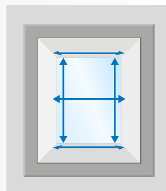
Figur 2. Montering i vindusramme/nisje.
